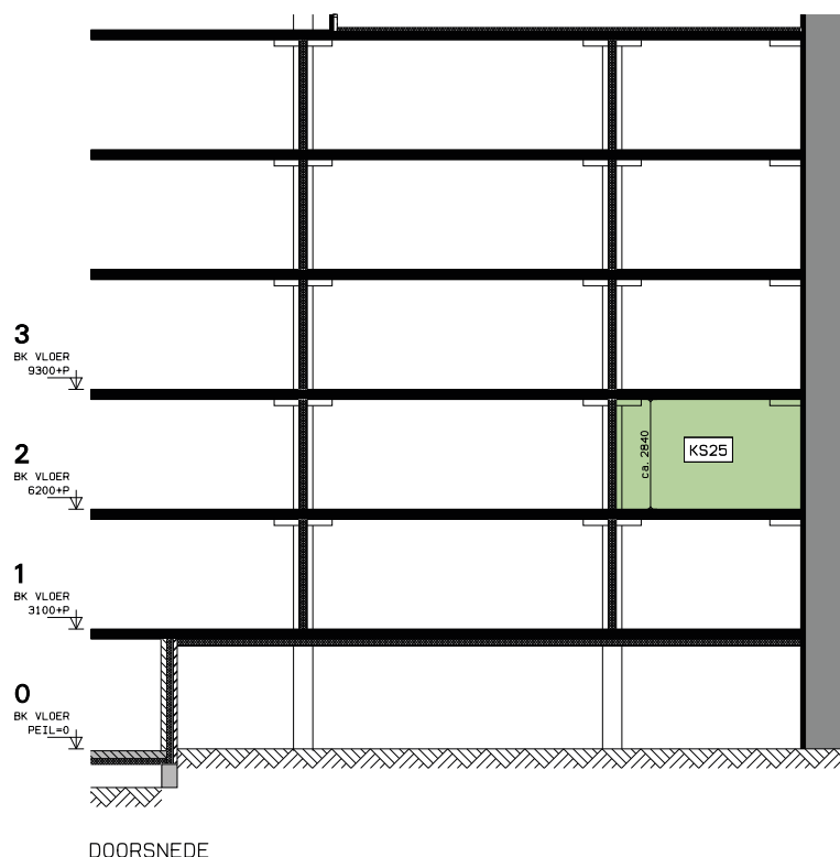
DOORSNEDE
