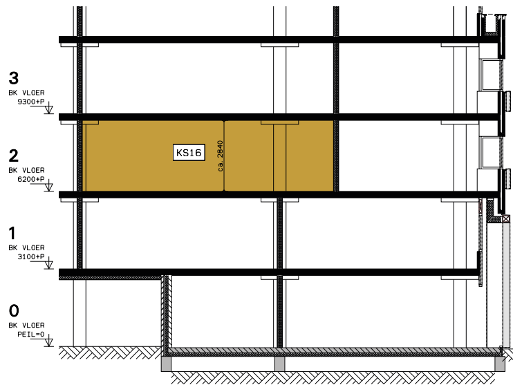
DOORSNEDE
